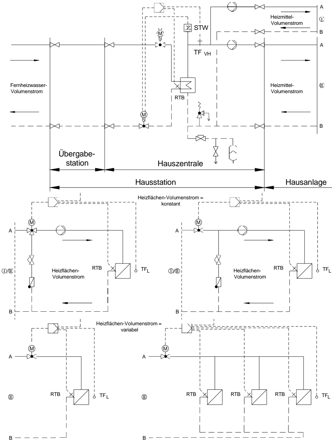
Bild 1: Hauszentrale-Raumluftheizung (RLH)
