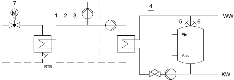
Speicher mit eingebauter Heizfläche
