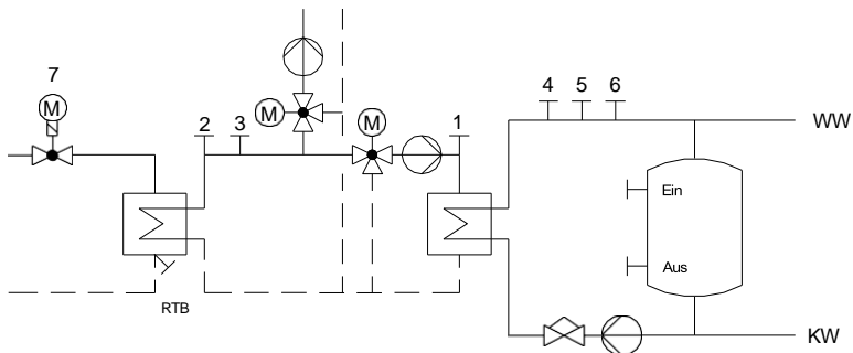
Speicherladesystem
