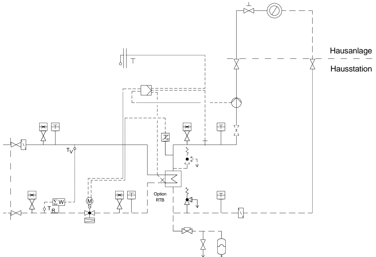
Bild 2: Hauszentrale-Raumheizung Prinzipschaltbild für den indirekten Anschluss
