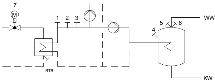
Speicherladesystem
